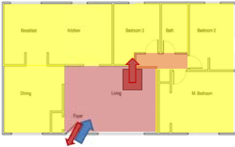
Figuur 4.14: Stromingspad rechtstreeks in en uit de brandruimte
